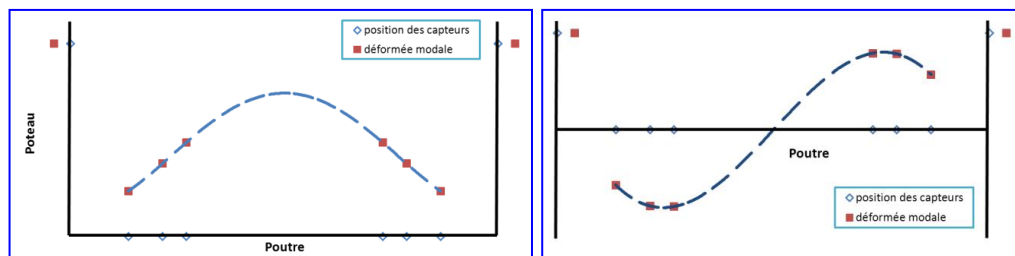
Figure 3. Déformées modales obtenues ; gauche à 73 Hz et droite à 195 Hz.
